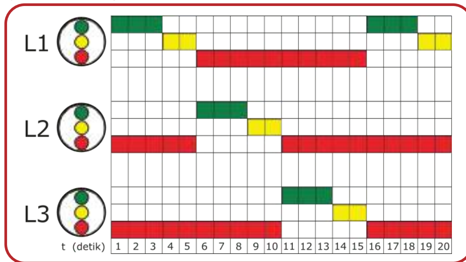
Gambar 2.10 Skema Diagram Waktu Lampu Rambu Lalu Lintas 1
